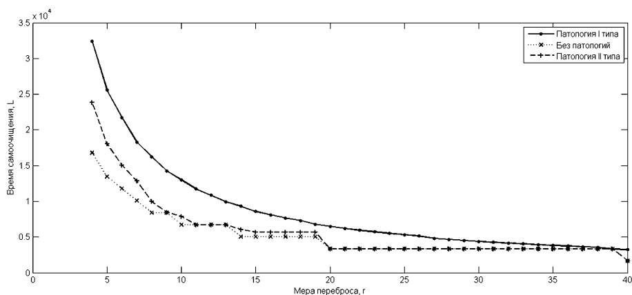
Рис. 1. График зависимости временной функции Шеннона от меры переброса.
